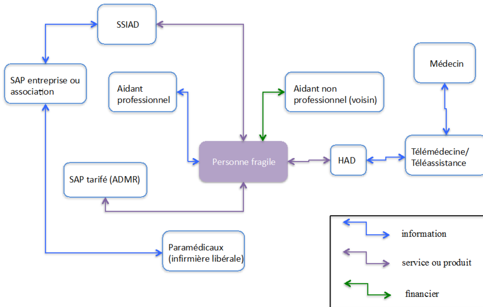
Figure 8 : Modèle d'interaction
